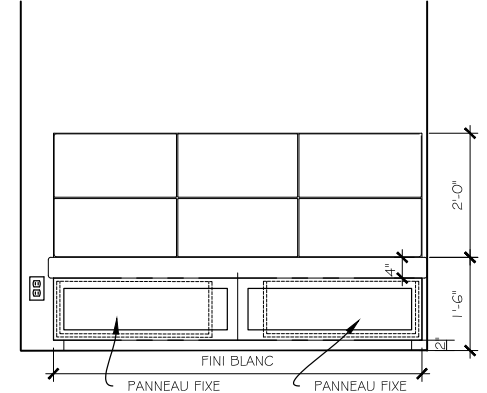
E3 ÉLÉVATION BANQUETTE ÉCH: 1/2" = 1'-0"
