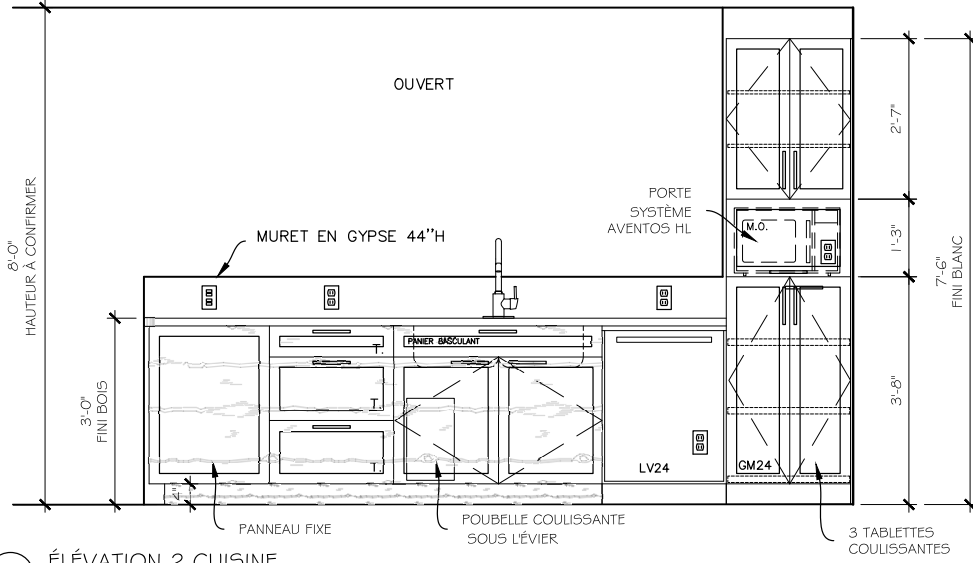
E2 ÉLÉVATION 2 CUISINE ÉCH: 1/2" = 1'-0"
