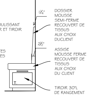
E4 PROFIL BANQUETTE ÉCH: 1/2" = 1'-0"
