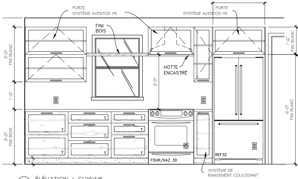
E1 ÉLÉVATION 1 CUISINE ÉCH: 1/2" = 1'-0"
