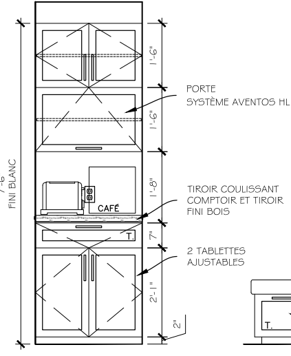
E5 ÉLÉVATION COIN CAFÉ ÉCH: 1/2" = 1'-0"
